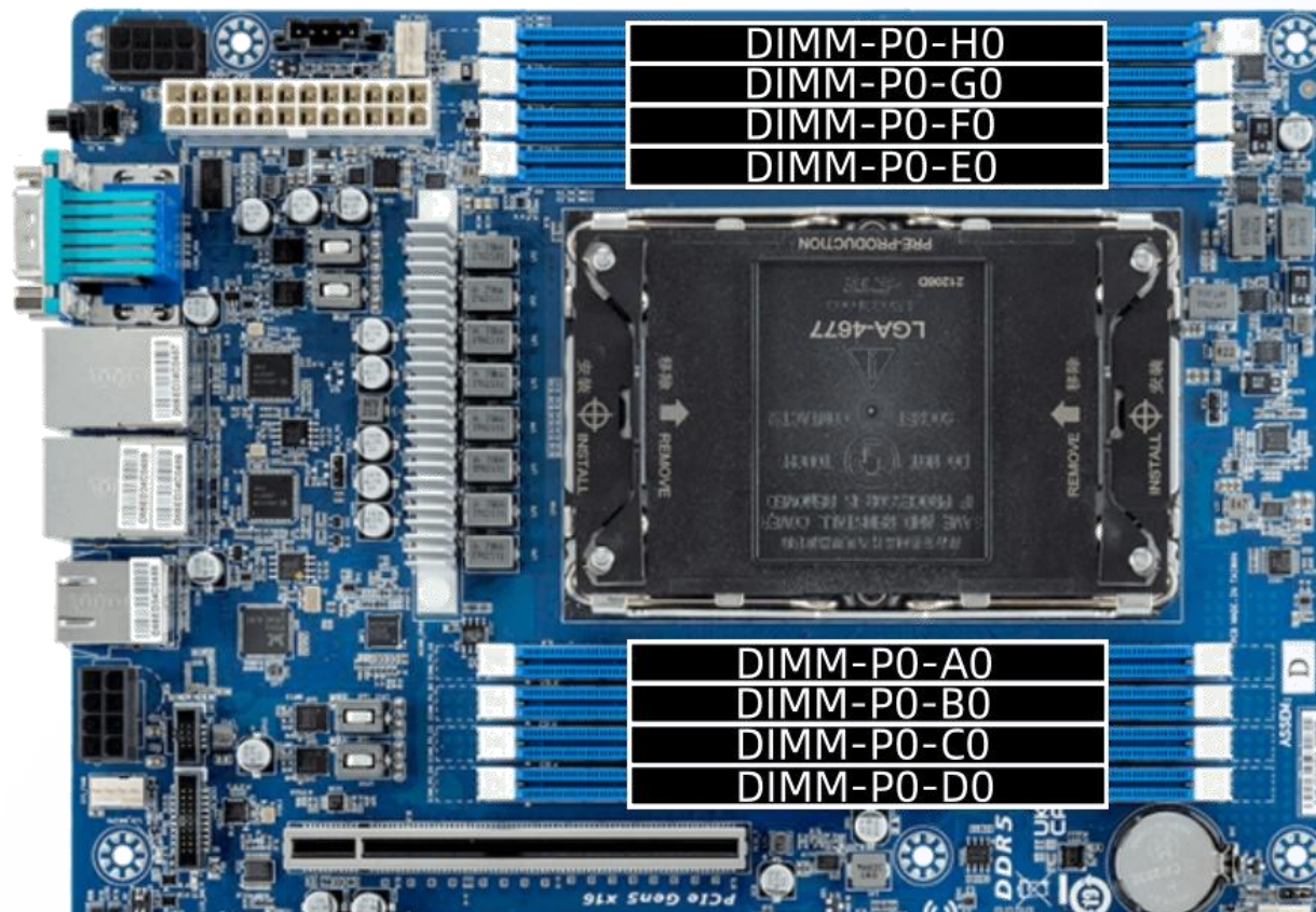
DIMM位置图
