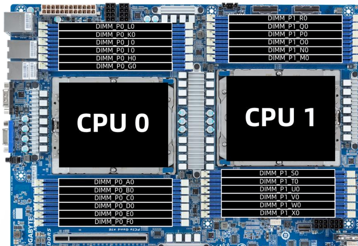
DIMM位置图
